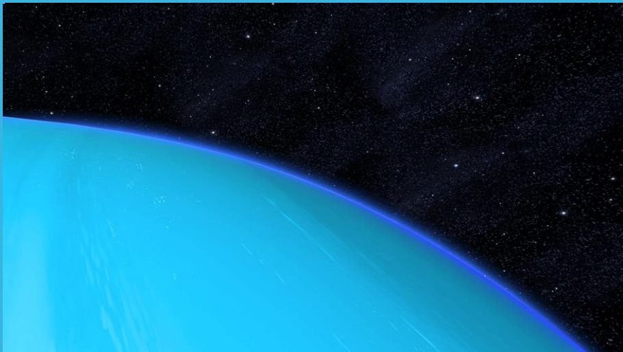
URAN
