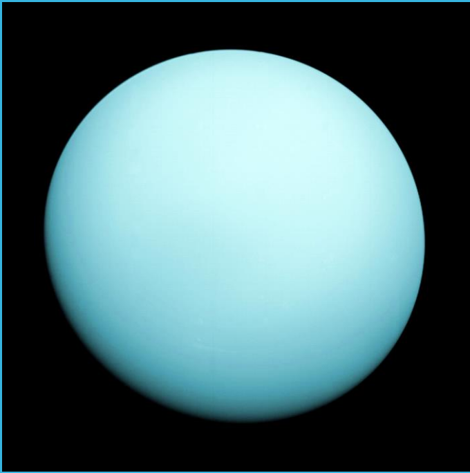
URAN
