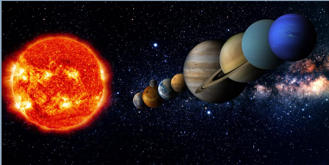
SUNČEV SUSTAV
