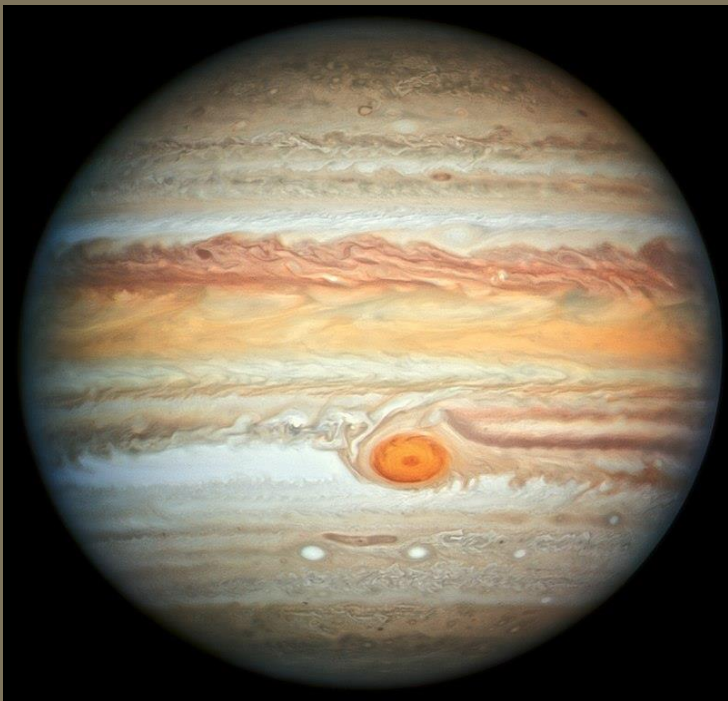
JUPITER
