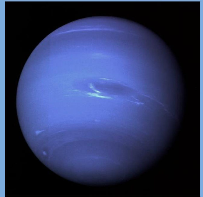
NEPTUN
