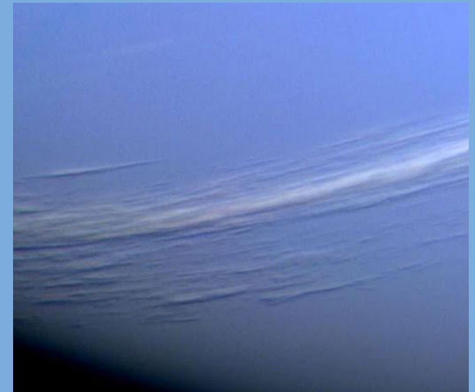
NEPTUN
